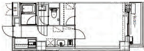
1K(29㎡)
